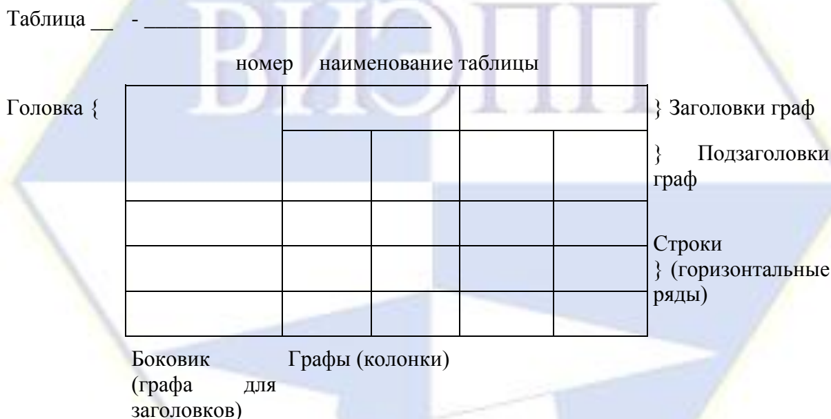
Рисунок 2 – Макет таблицы
