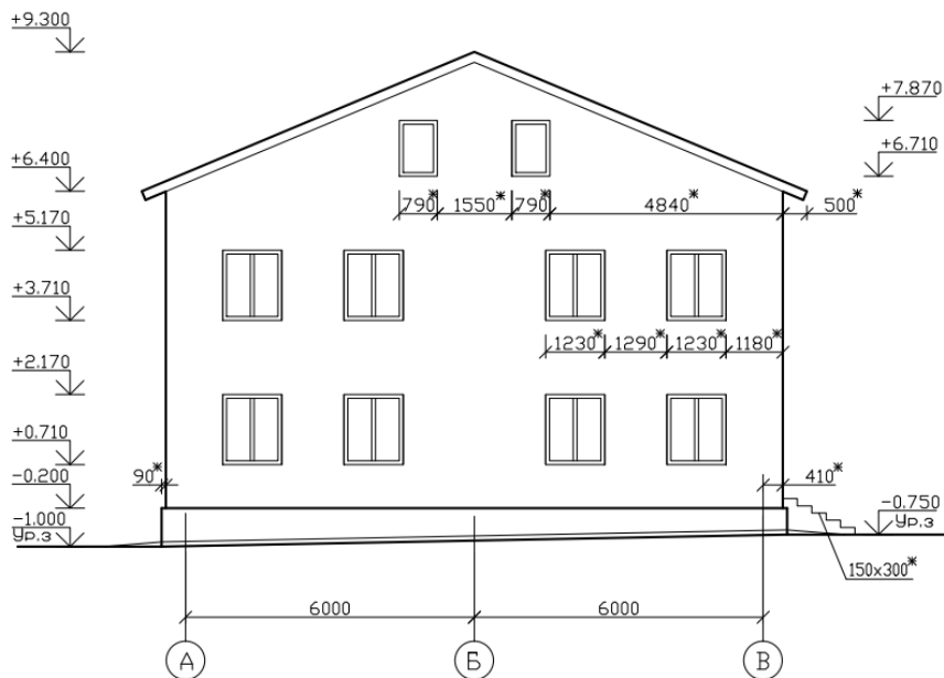
Фасад А-В
